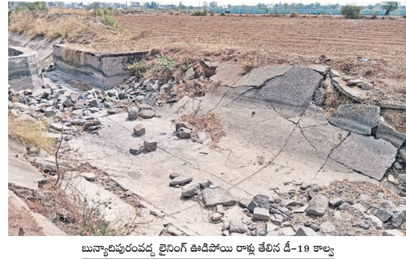
బున్యాదిపురం వద్ద లైనింగ్ ఊడిపోయి రాళ్లు తేలిన డి-19 కాల్వ
